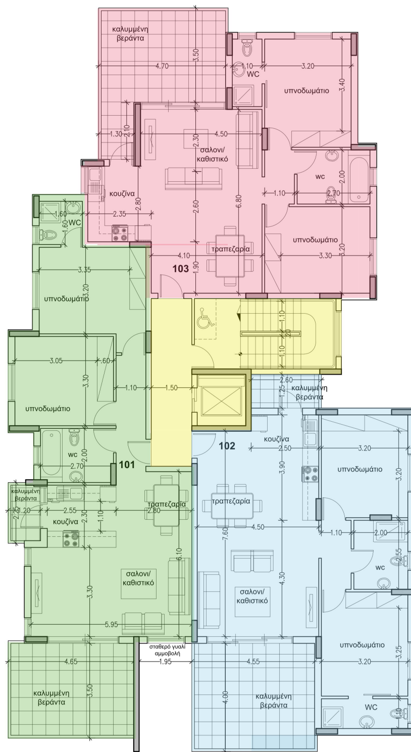
ΚΑΤΟΨΗ 1ου ΟΡΟΦΟΥ
