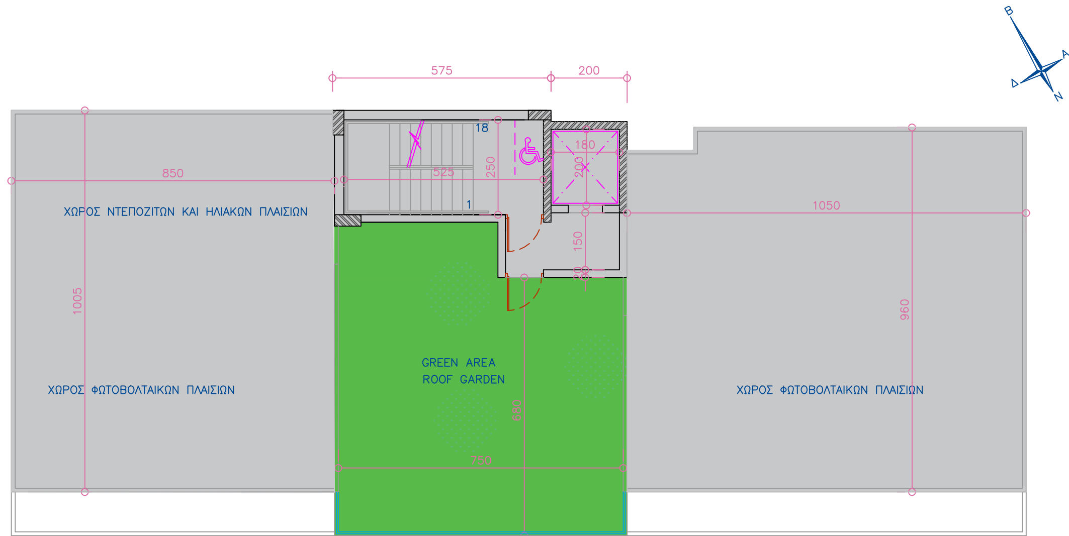
ΚΑΤΟΨΗ ΤΑΡΑΤΣΙΑΣ BLOCK C
