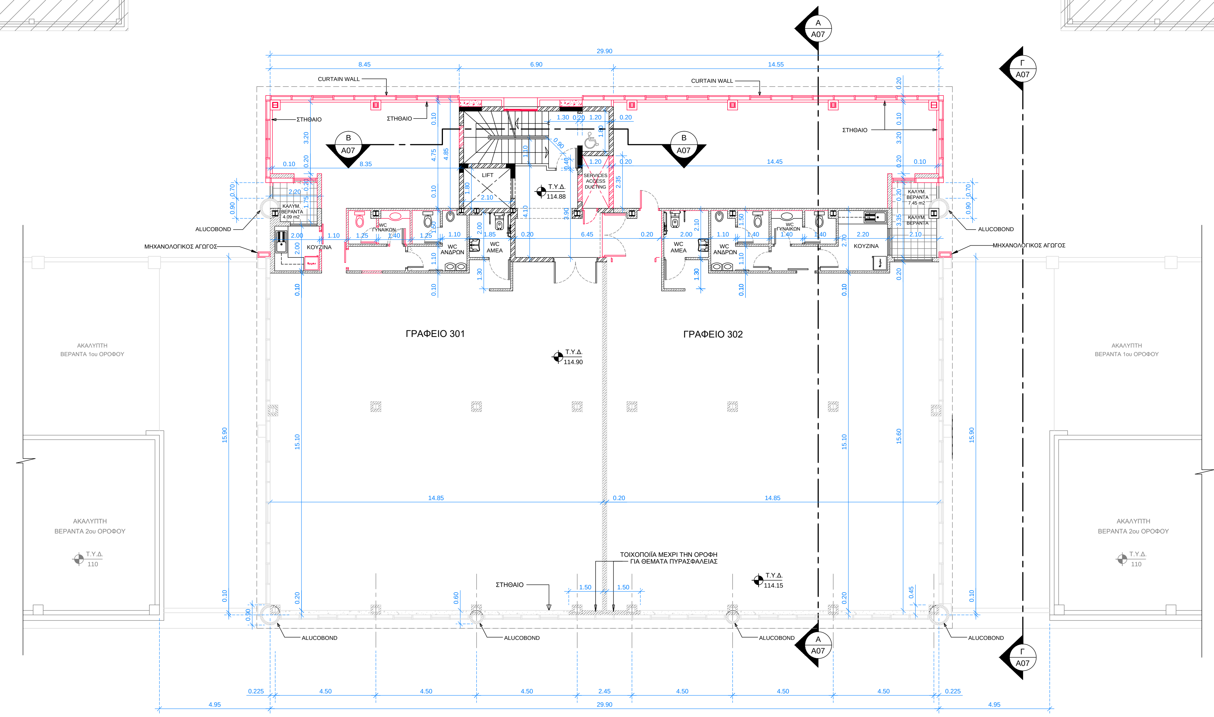
BLOCK C ΚΑΤΟΨΗ 3ου ΟΡΟΦΟΥ - ΕΠΕΚΤΑΣΗ ΓΡΑΦΕΙΩΝ ΚΛ. 1:100
