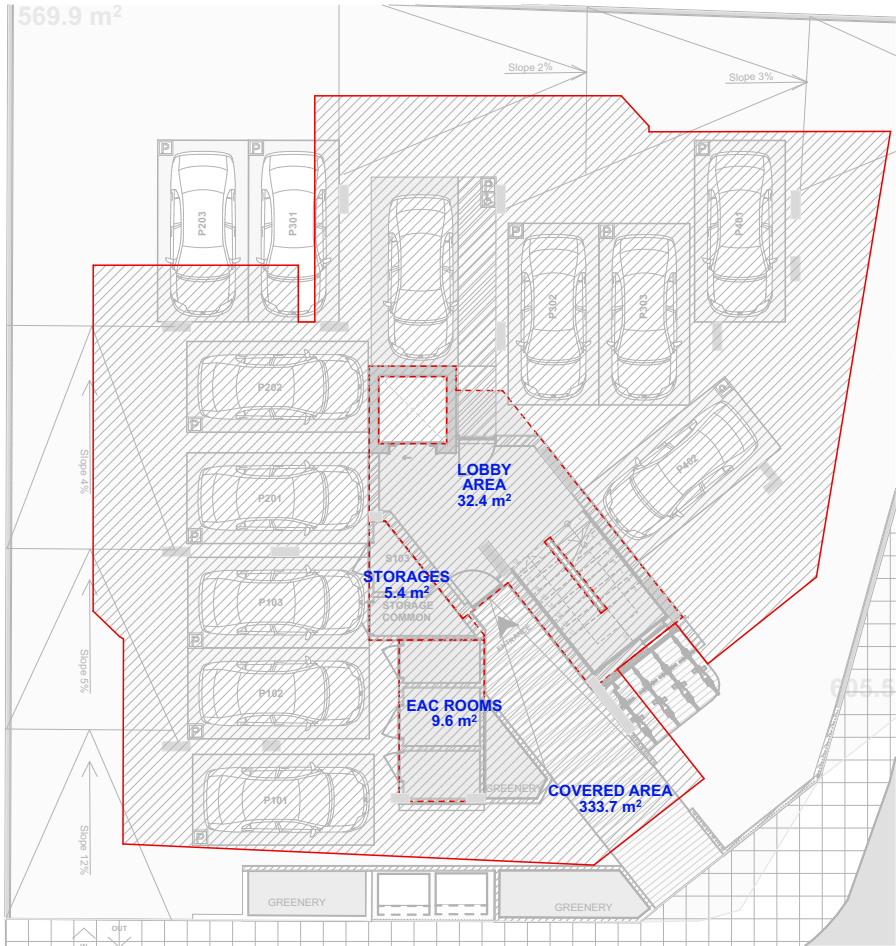
ΙΣΟΓΕΙΟ ΕΜΒΑΔΟΜΕΤΡΗΣΗ - ΚΛΙΜΑΚΑ 1:200
