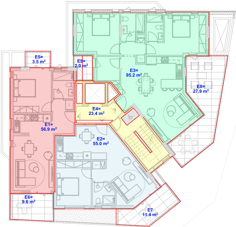
1 ος ΟΡΟΦΟΣ ΕΜΒΑΔΟΜΕΤΡΗΣΗ - ΚΛΙΜΑΚΑ 1:200 E01 + E02 + E03 + E04 = 56.9 + 55.0 + 95.2 + 23.4 = 230.5 m²
