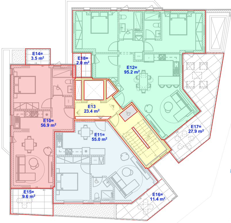
2 ος ΟΡΟΦΟΣ ΕΜΒΑΔΟΜΕΤΡΗΣΗ - ΚΛΙΜΑΚΑ 1:200 E10 + E11 + E12 + E13 = 56.9 + 55.0 + 95.2 + 23.4 = 230.5 m²
