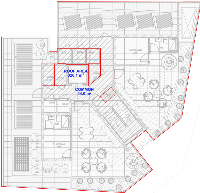
ROOF GARDEN ΕΜΒΑΔΟΜΕΤΡΗΣΗ - ΚΛΙΜΑΚΑ 1:200
