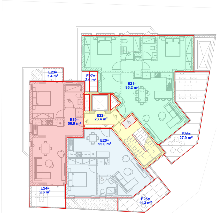
3 ος ΟΡΟΦΟΣ ΕΜΒΑΔΟΜΕΤΡΗΣΗ - ΚΛΙΜΑΚΑ 1:200 E19 + E20 + E21 + E22 = 56.7 + 55.0 + 95.2 + 23.4 = 230.5 m²
