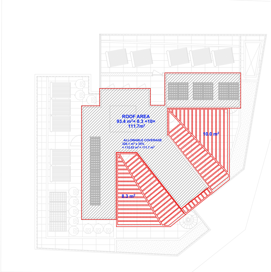
ΟΡΟΦΗ ΕΜΒΑΔΟΜΕΤΡΗΣΗ - ΚΛΙΜΑΚΑ 1:200
