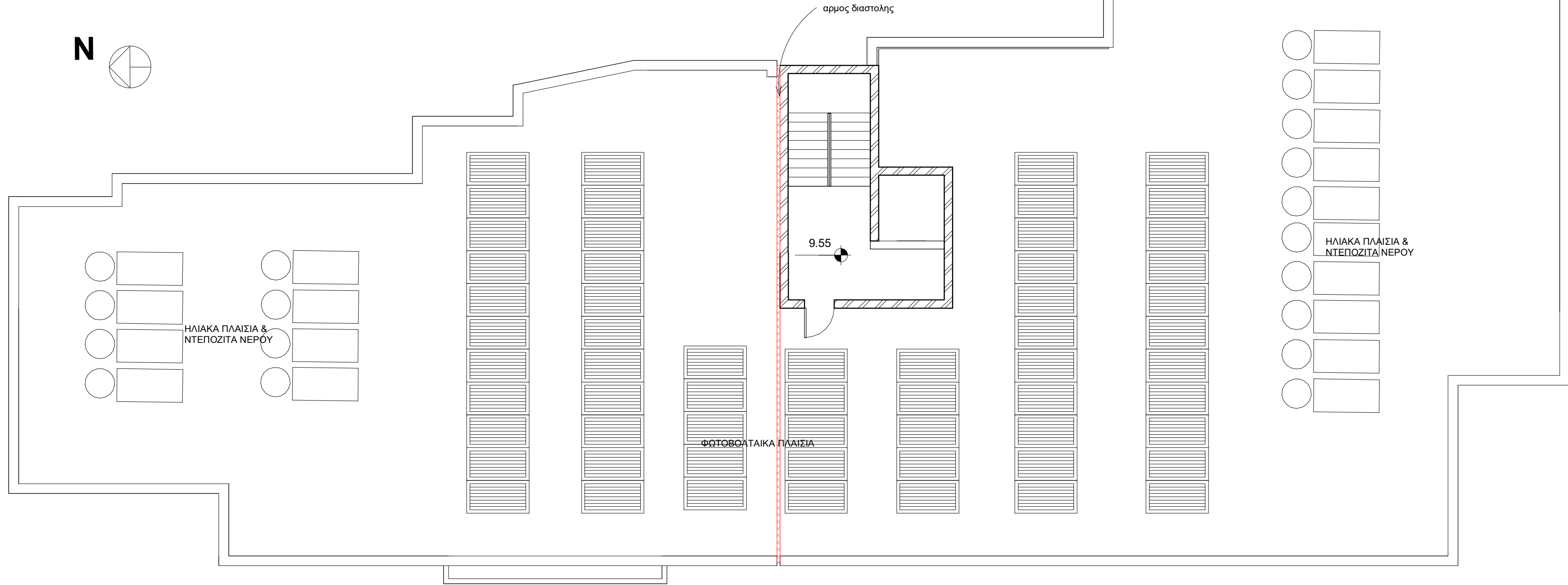
1 Roof 1 : 100
