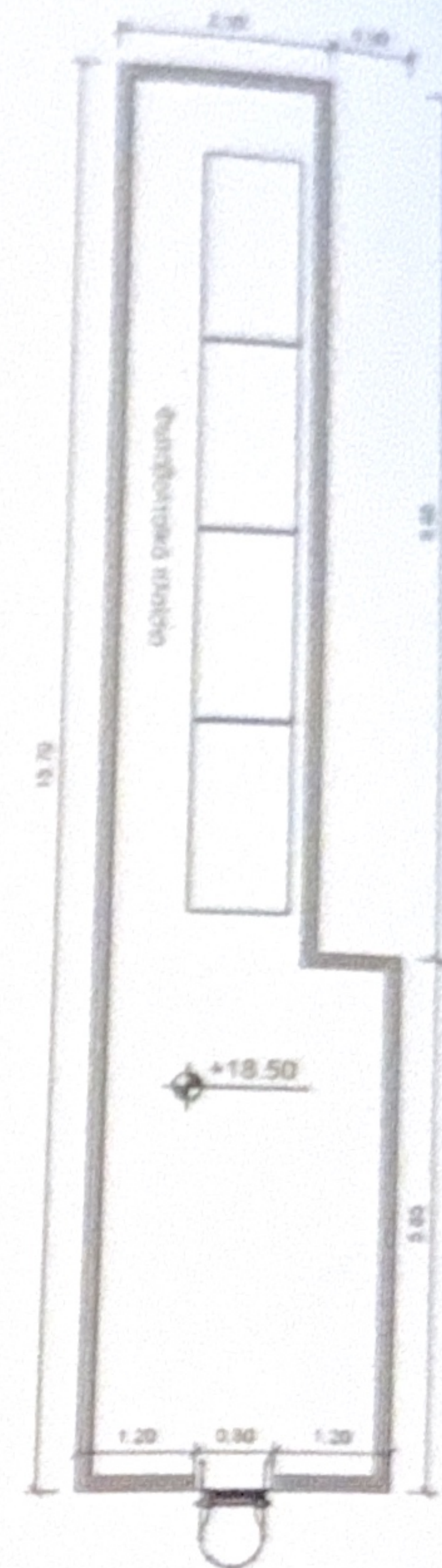
ΚΑΤΩΦΗ ΟΡΟΦΗΣ ΚΛΙΜΑΚΟΣΤΑΣΙΟΥ
