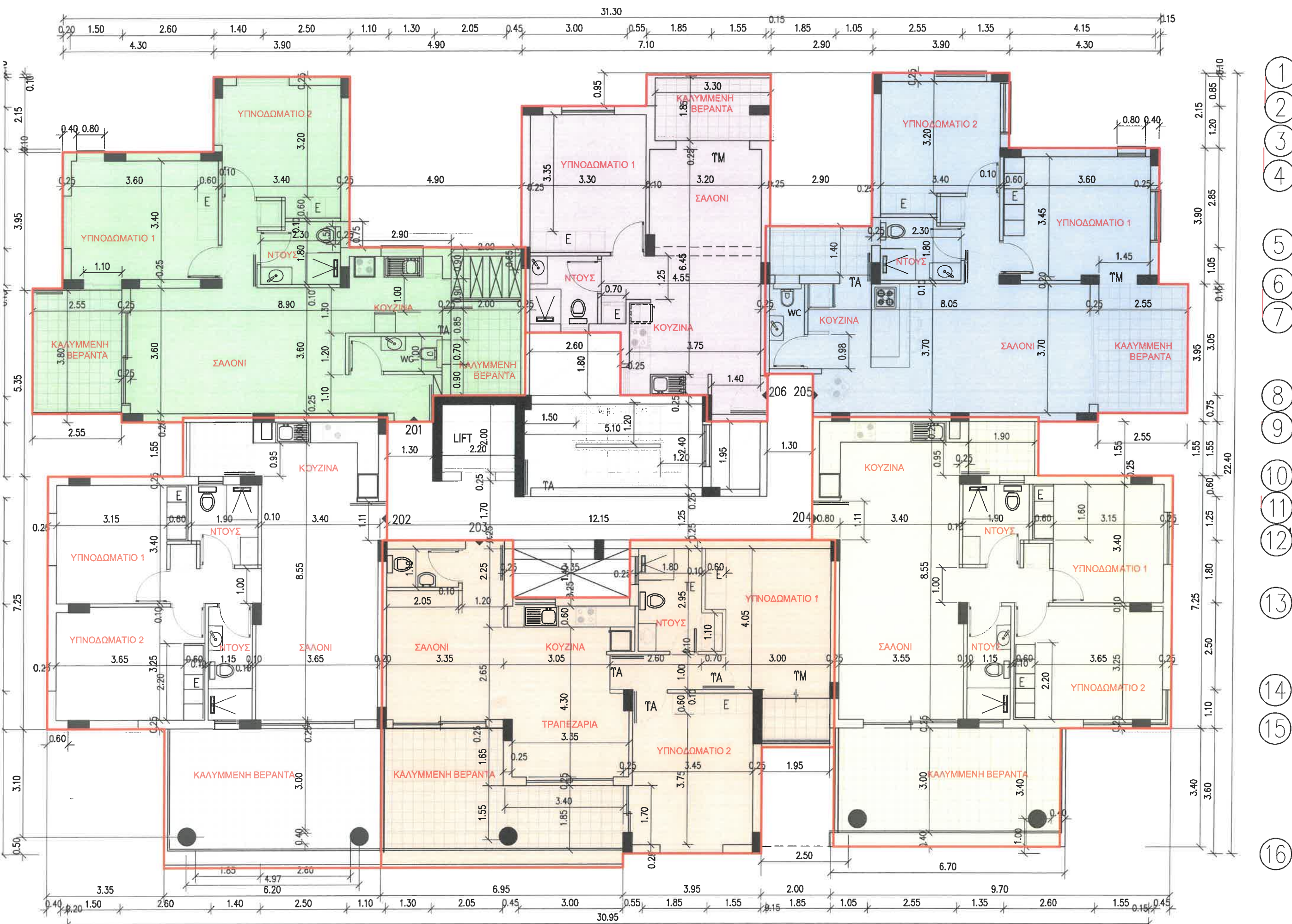
ΚΑΤΟΨΗ 2ου ΟΡΟΦΟΥ
