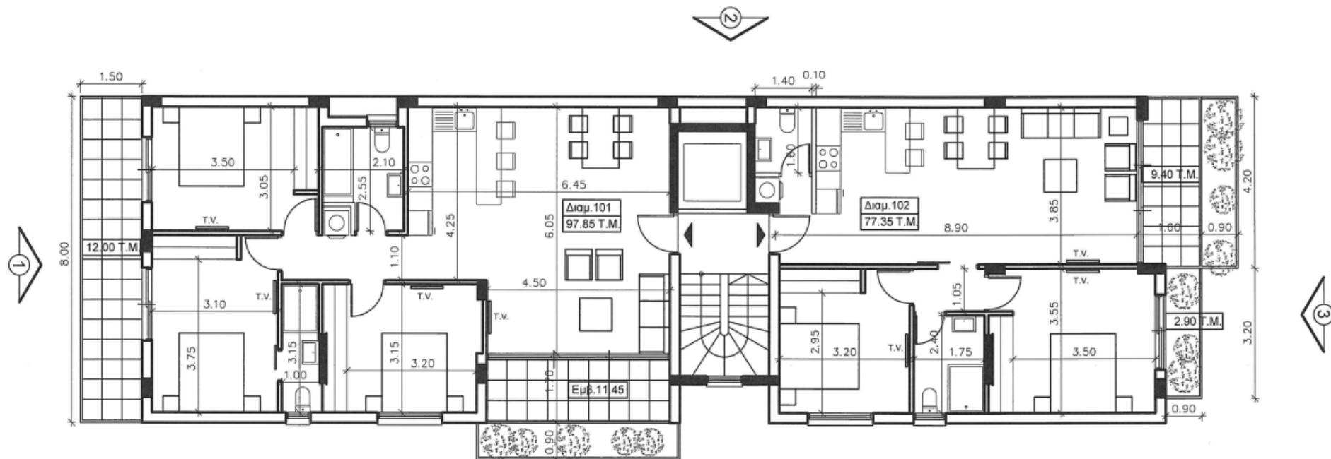
ΚΑΤΟΨΗ 1ου ΟΡΟΦΟΥ ΚΛΙΜΑΚΑ 1:100
