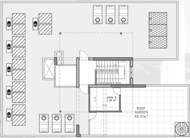
ΚΑΤΟΨΗ ΟΡΟΦΗΣ
