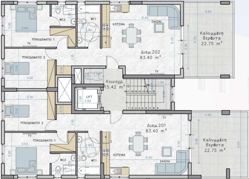
ΚΑΤΟΨΗ 2 ου ΟΡΟΦΟΥ
