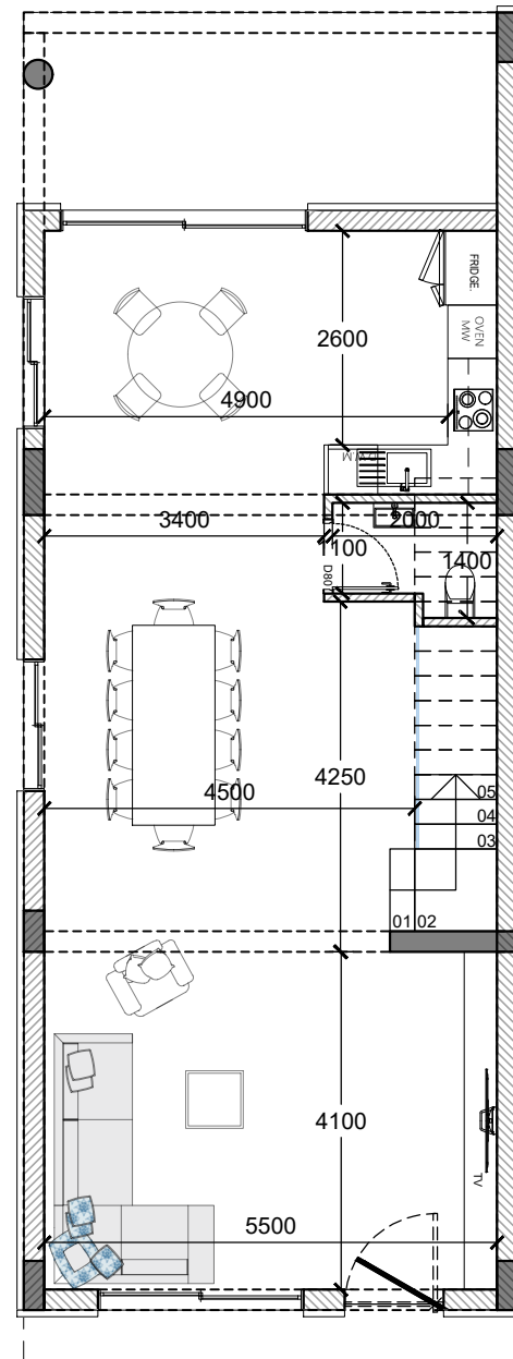
ΚΑΤΟΨΗ ΙΣΟΓΕΙΟΥ
