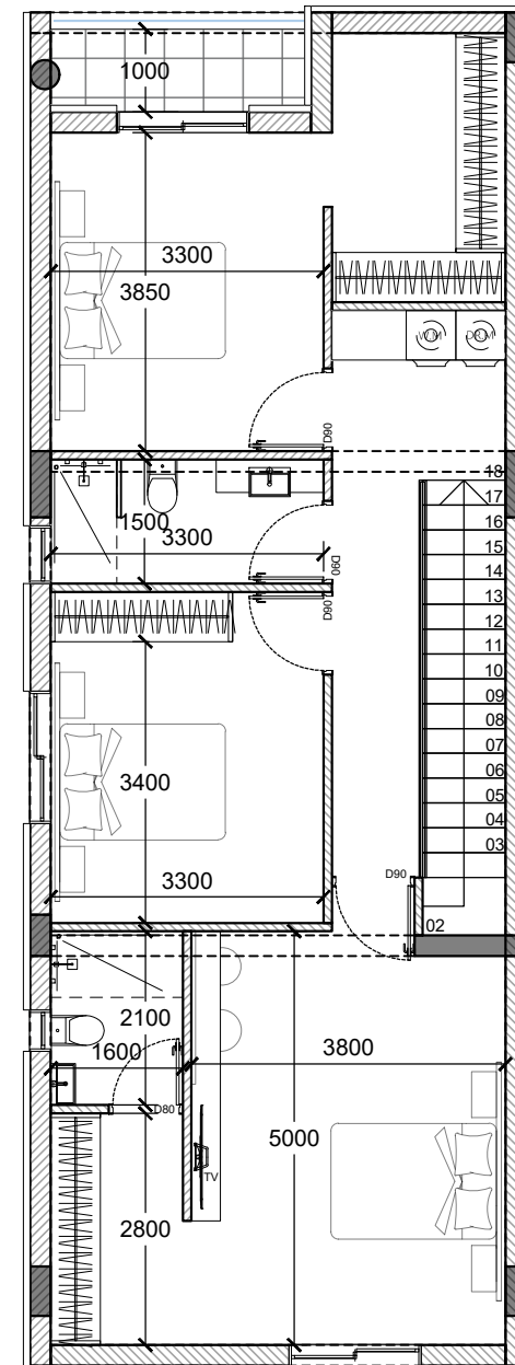
ΚΑΤΟΨΗ ΟΡΟΦΟΥ
