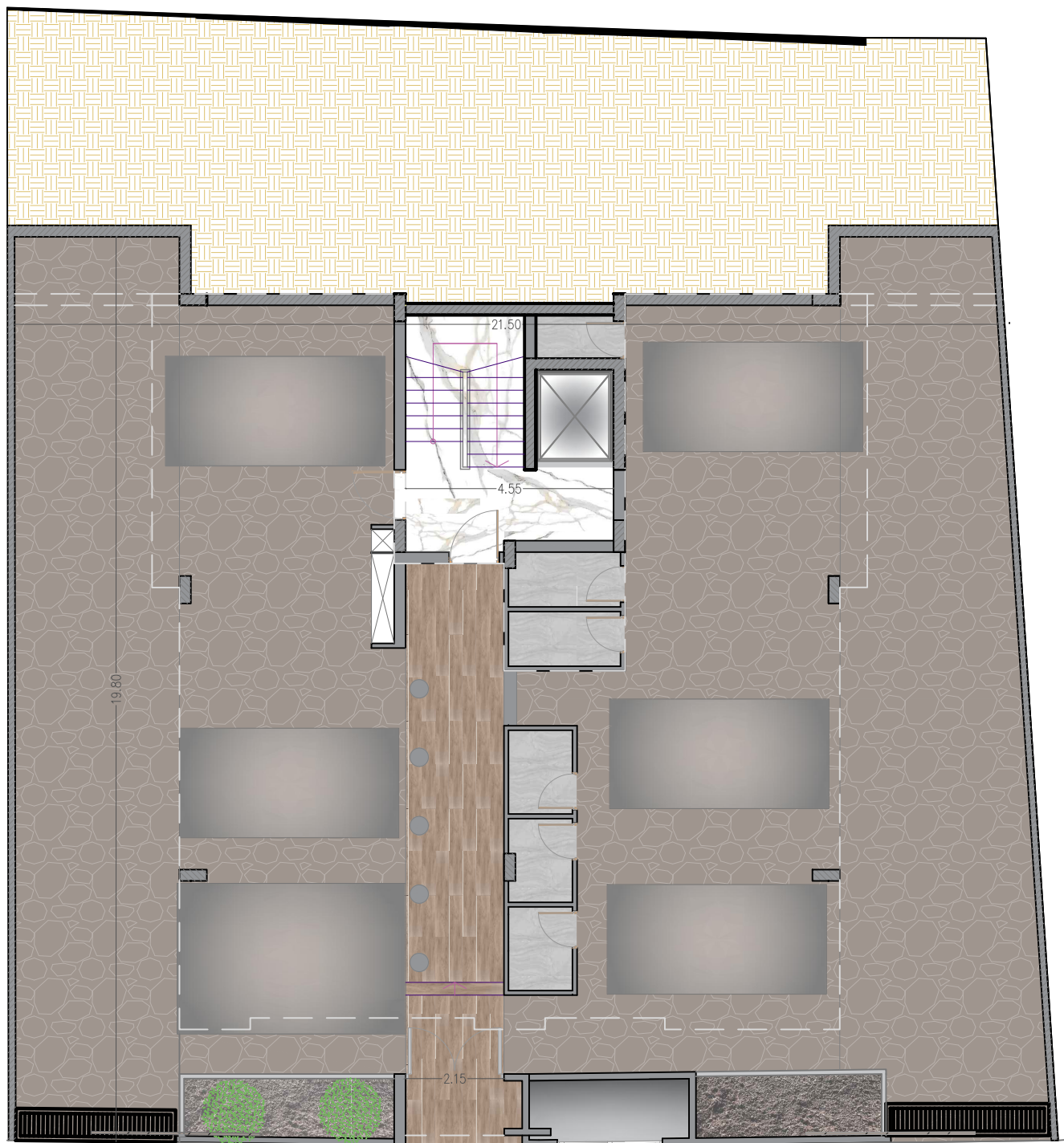
ΚΑΤΟΨΗ ΙΣΟΓΕΙΟΥ
