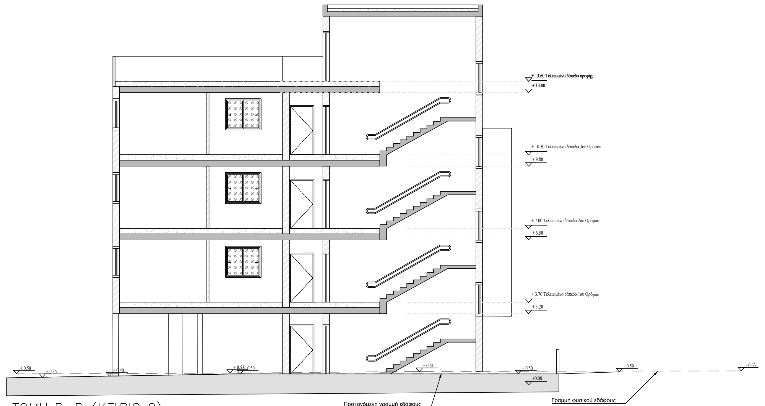
ΤΟΜΗ Β-Β (ΚΤΙΡΙΟ 2)
