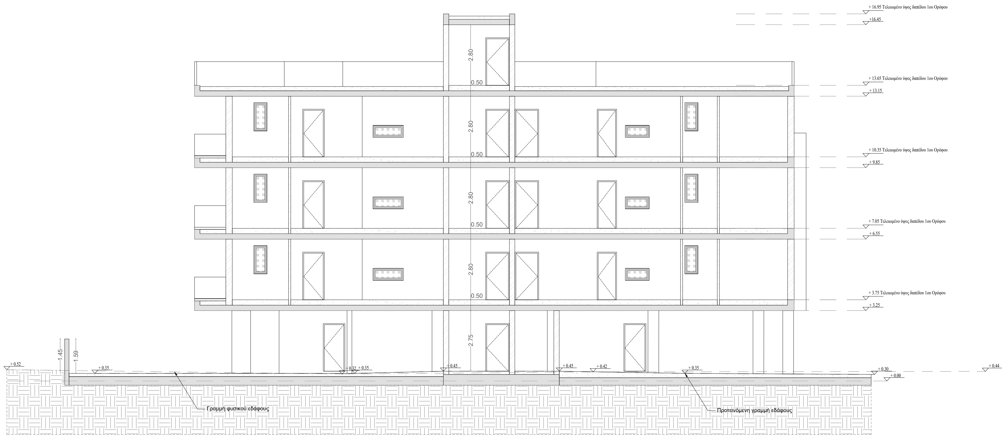
ΚΤΙΡΙΟ 1 ΤΟΜΗ Α-Α
