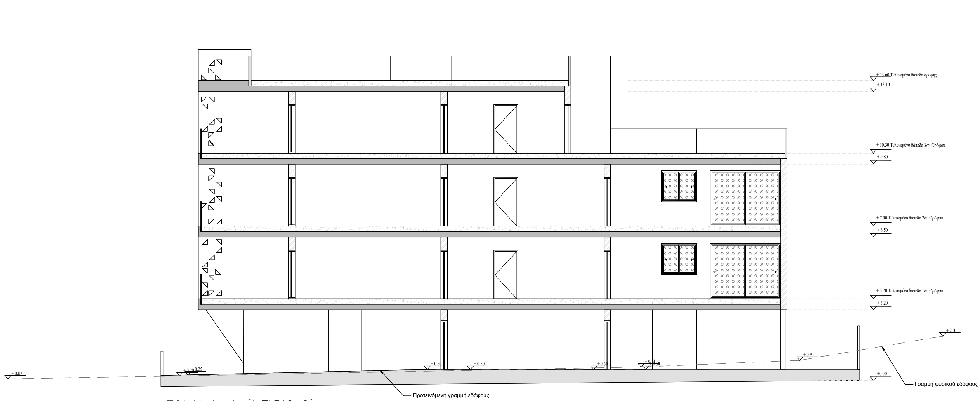
ΤΟΜΗ Α-Α (ΚΤΙΡΙΟ 2)
