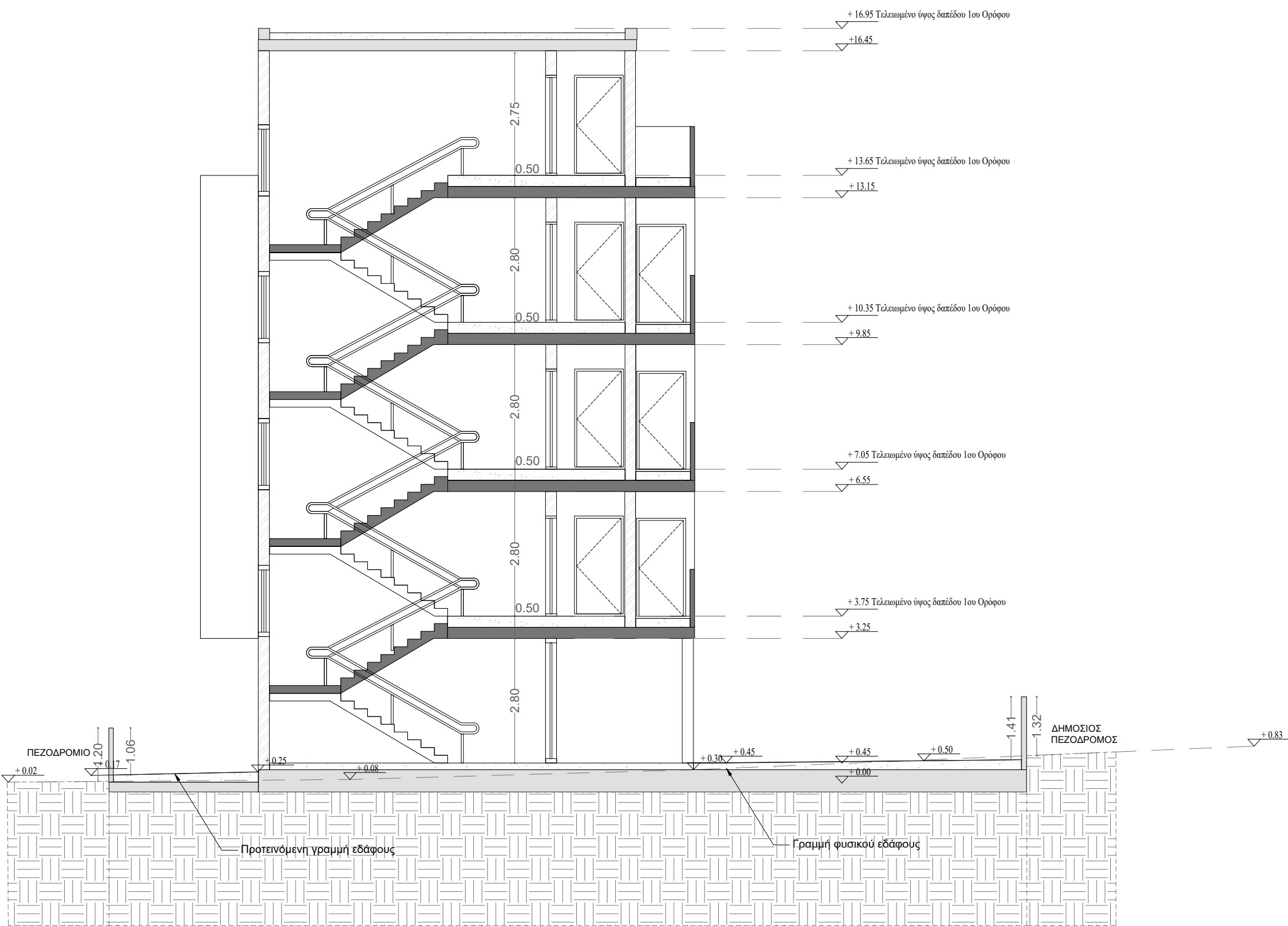
ΚΤΙΡΙΟ 1 ΤΟΜΗ Β-Β
